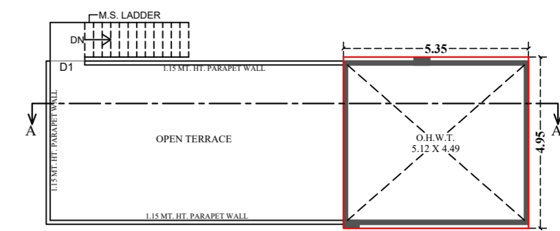
O.H.W.T. PLAN OPEN TERRACE
