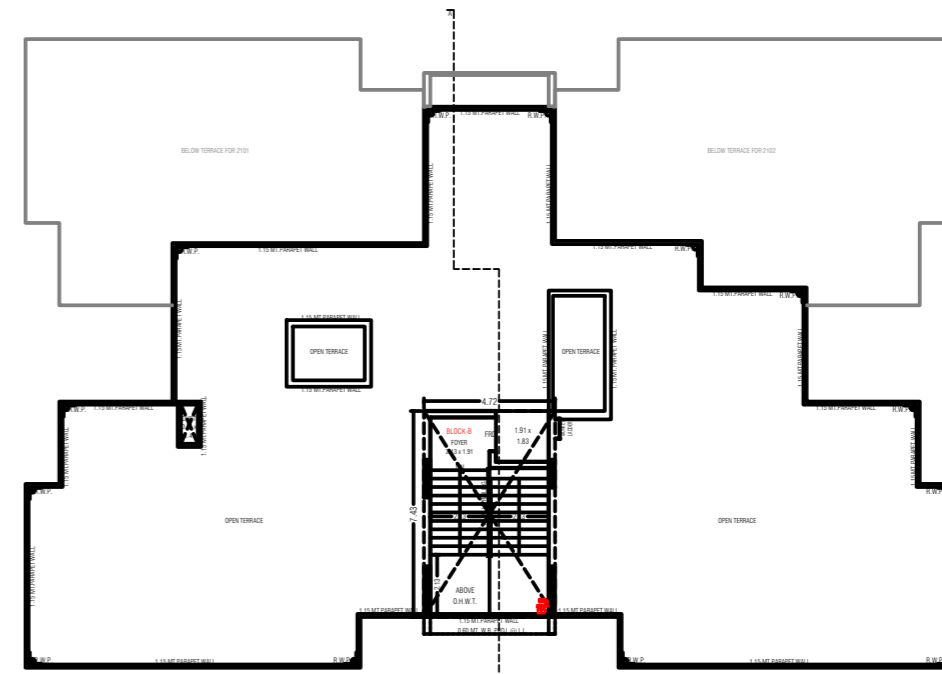
OPEN TERRACE PLAN(STAIR CABIN, O.H.W.T.)
