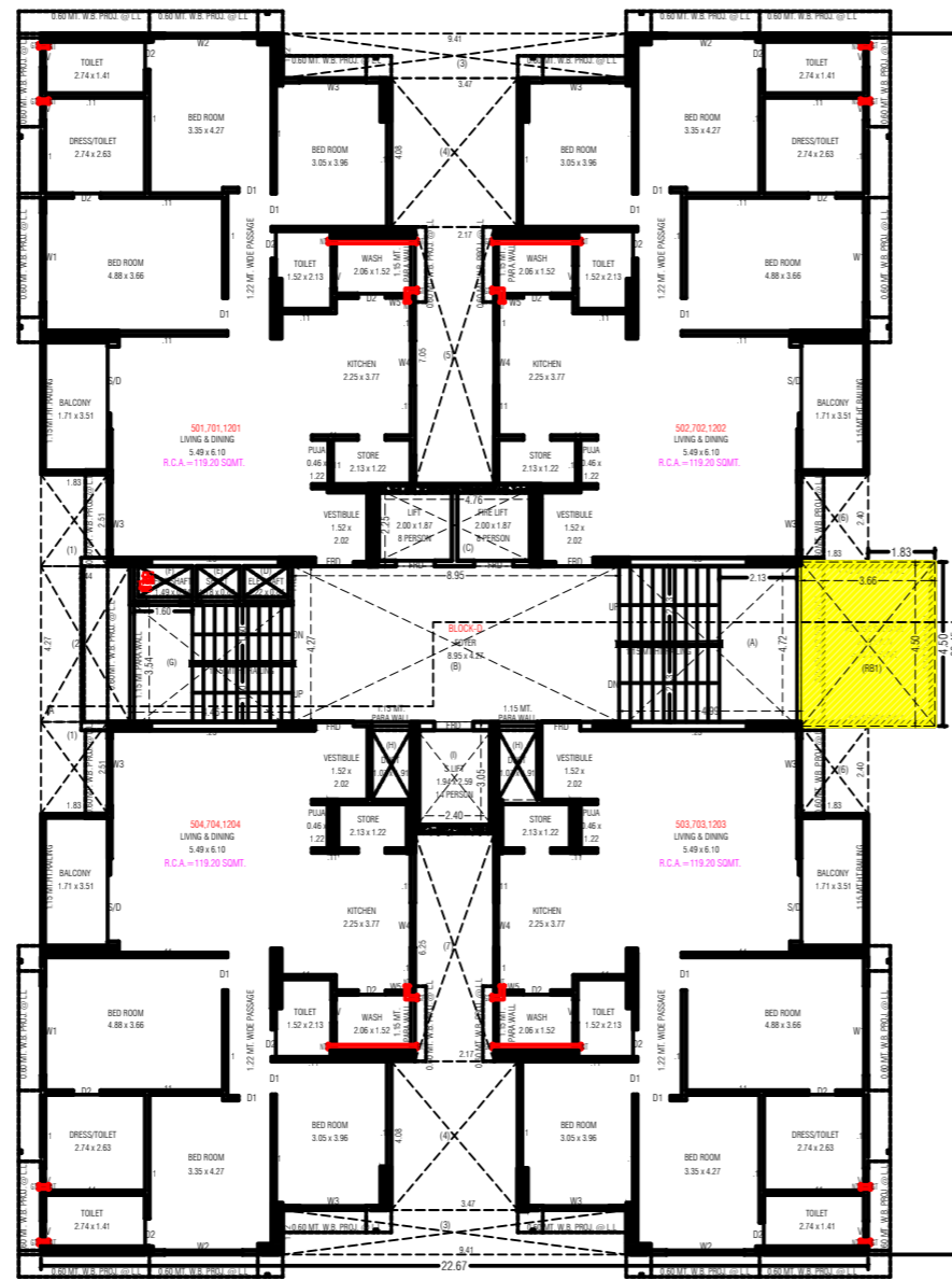
5TH.FL.,7TH.FL.,12TH.FLOOR PLAN
