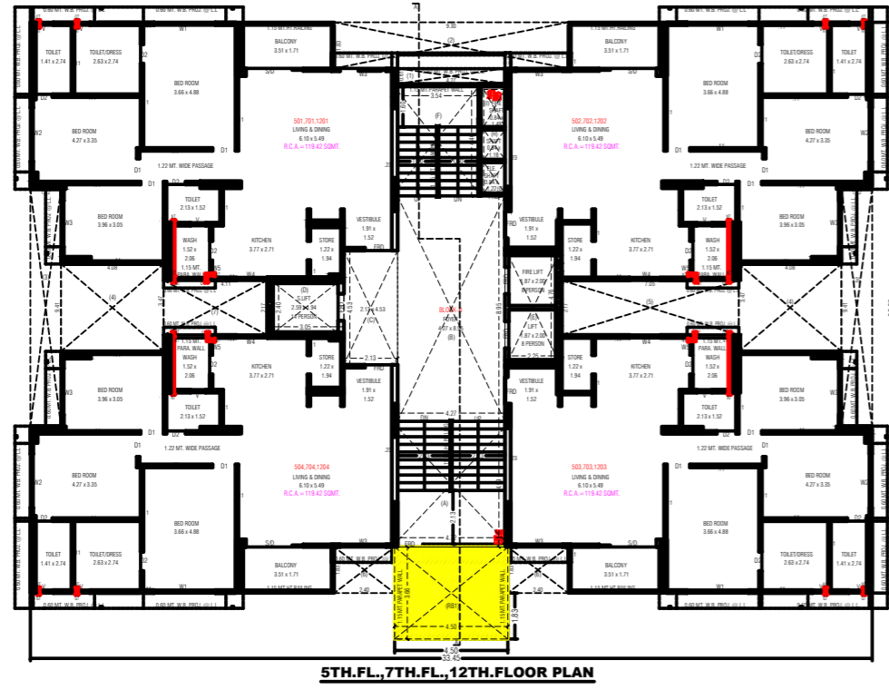
5TH.FL., 7TH.FL., 12TH.FLOOR PLAN
